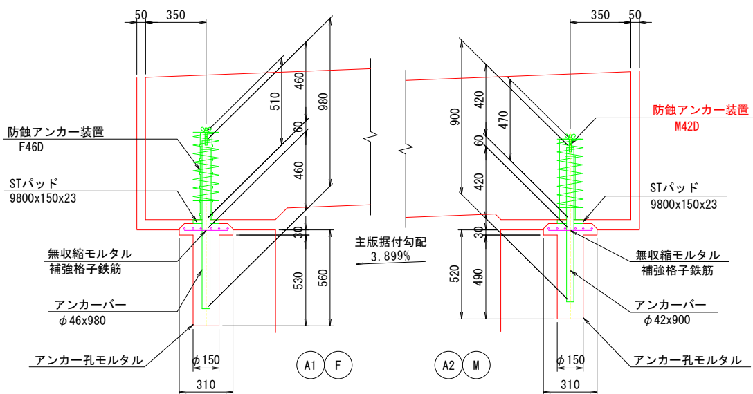
アンカー側面図
