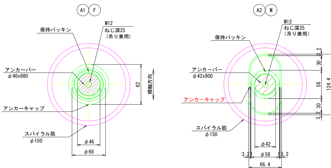
アンカー断面図
